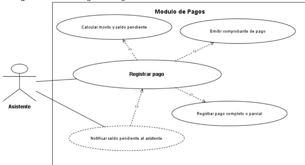
Figura 10: CU-04 Registrar Pago
