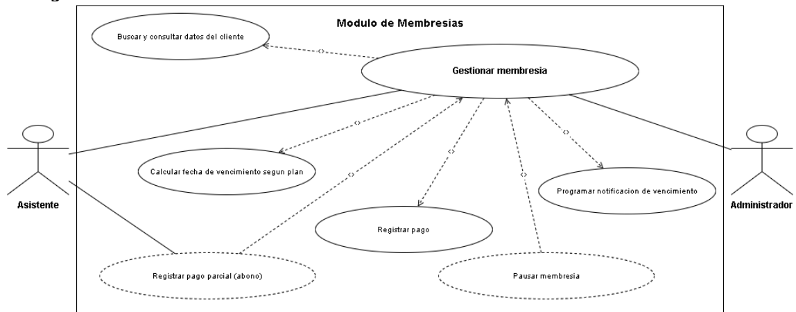
Figura 8: CU-02 Gestionar Membresia
