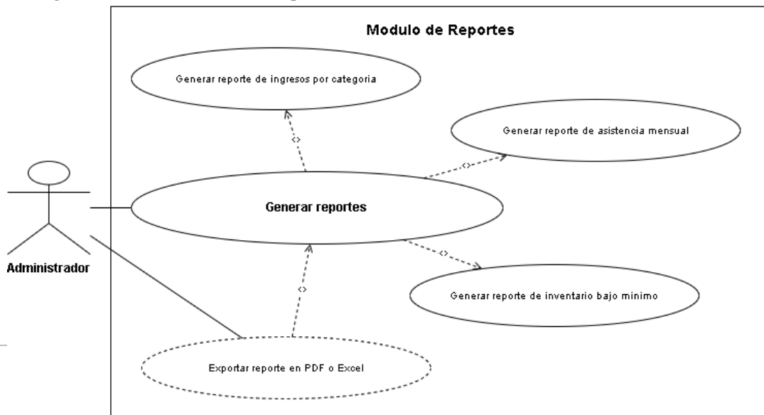
Figura 16: CU-10 Generar Reportes
