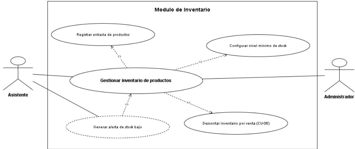
Figura 11: CU-05 Gestionar Inventario de Productos
