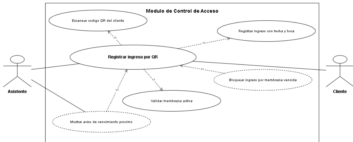
Figura 9: CU-03 Registrar Ingreso por QR
