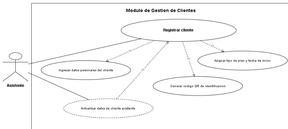
Figura 7: CU-01 Registrar Cliente
